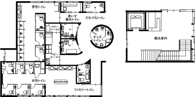
1F 図面
