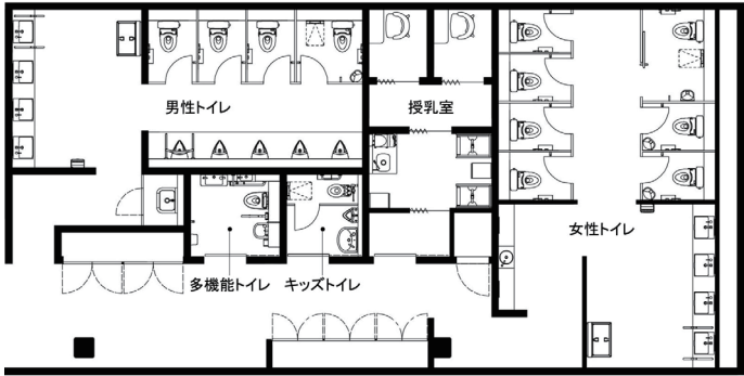
トイレ図面
