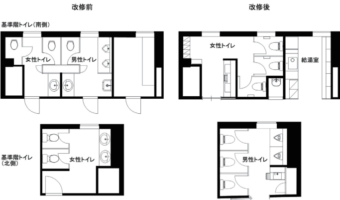
基準階 トイレ図面
