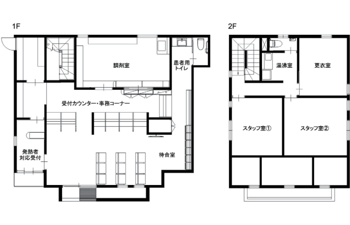
メディポリ薬局図面
