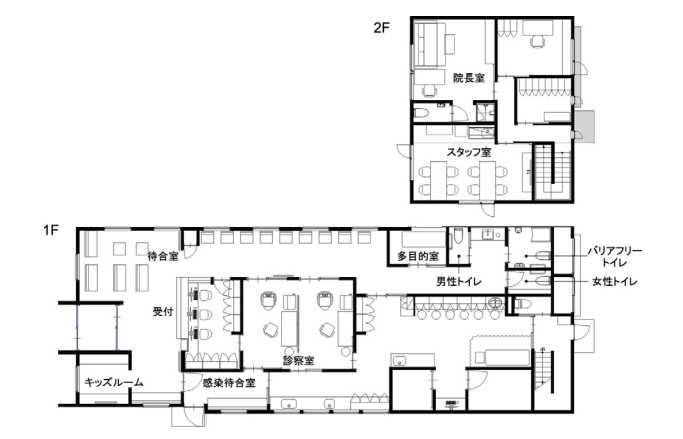
みみ はな のど たけだみクリニック図面
