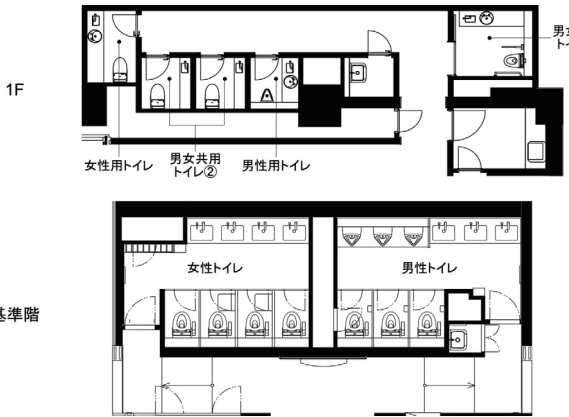
トイレ図面
