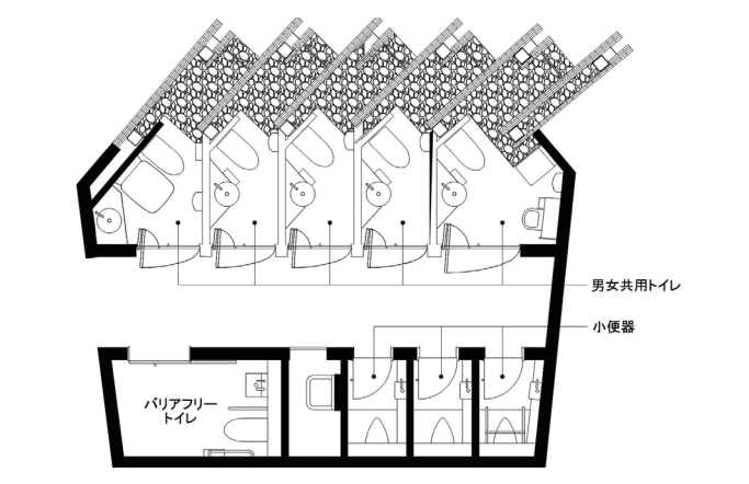
ファクトリーエリア トイレ図面
