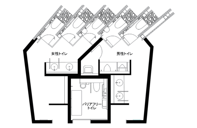
ファーム・プラントエリア トイレ図面
