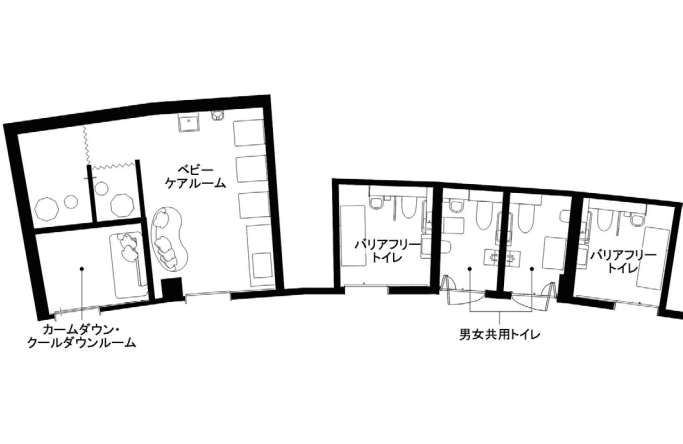
外周通路 トイレ図面
