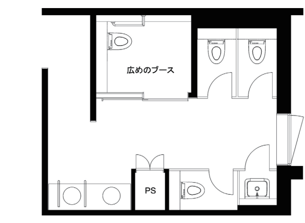
1F 男女共用トイレ図面
