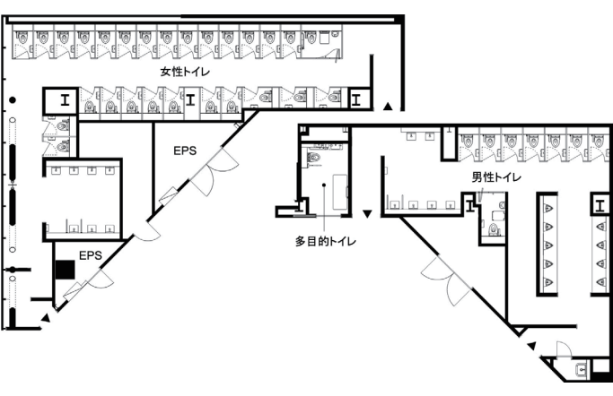
メインアリーナトイレ図面
